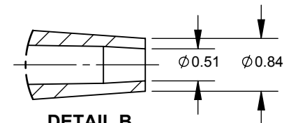
DETAIL B SCALE: 12 : 1
