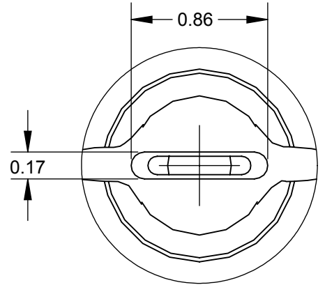
DETAIL B SCALE: 30 : 1
