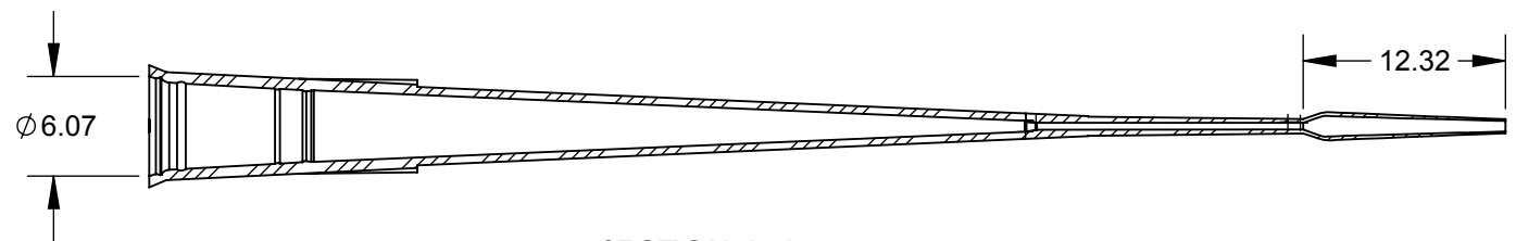
SECTION A-A SCALE: 2 : 1
