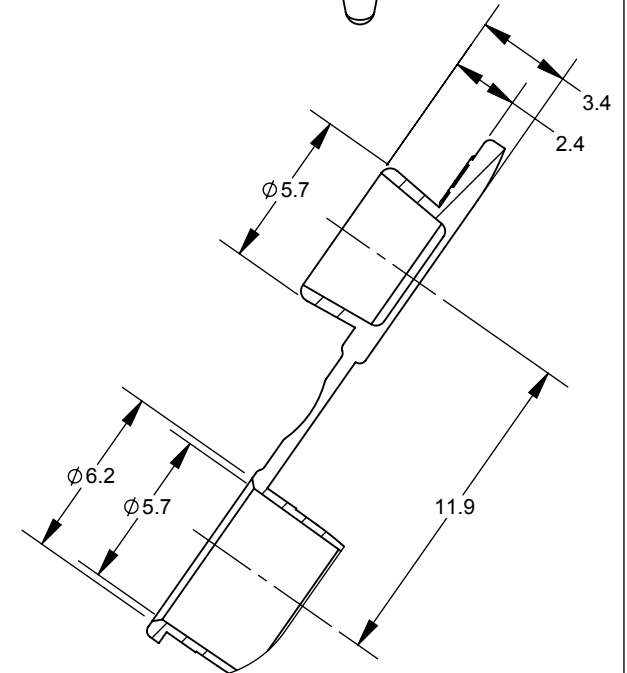
DETAIL B SCALE: 3.7 : 1 TYP
