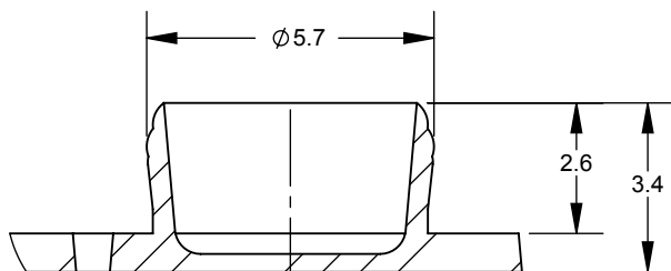
DETAIL B SCALE: 6 : 1 TYP
