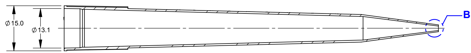
SECTION A-A
