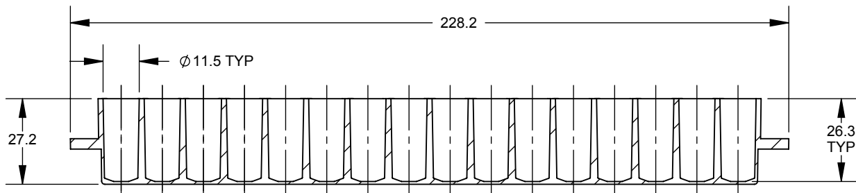
SECTION A-A SCALE: 0.6 : 1
