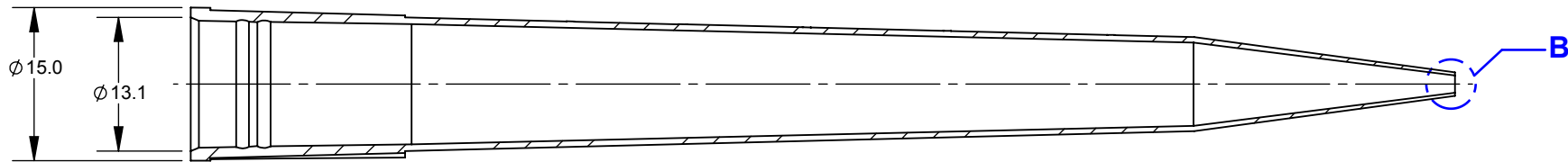
SECTION A-A
