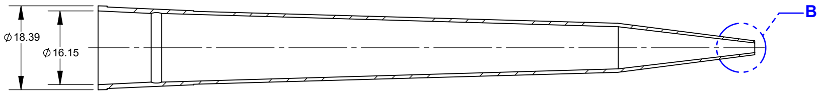
SECTION A-A SCALE: 1.2 : 1
