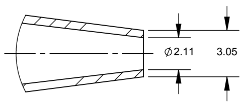
DETAIL B SCALE: 4 : 1
