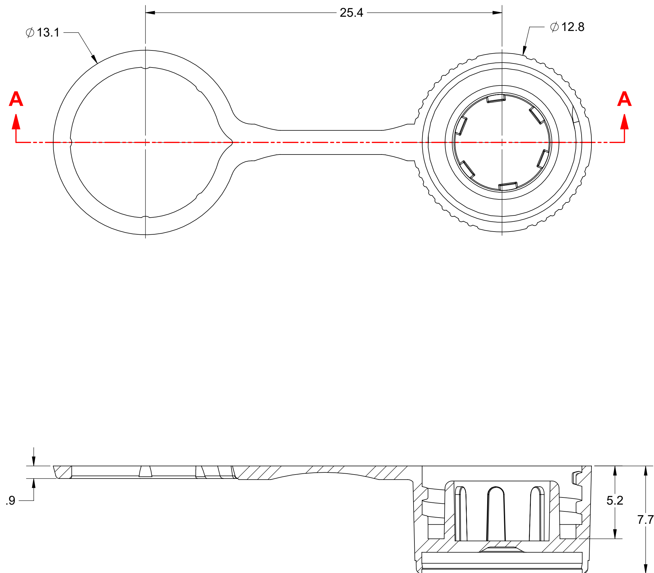
SECTION A-A
