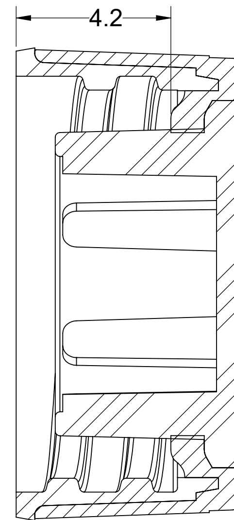
SECTION A-A
