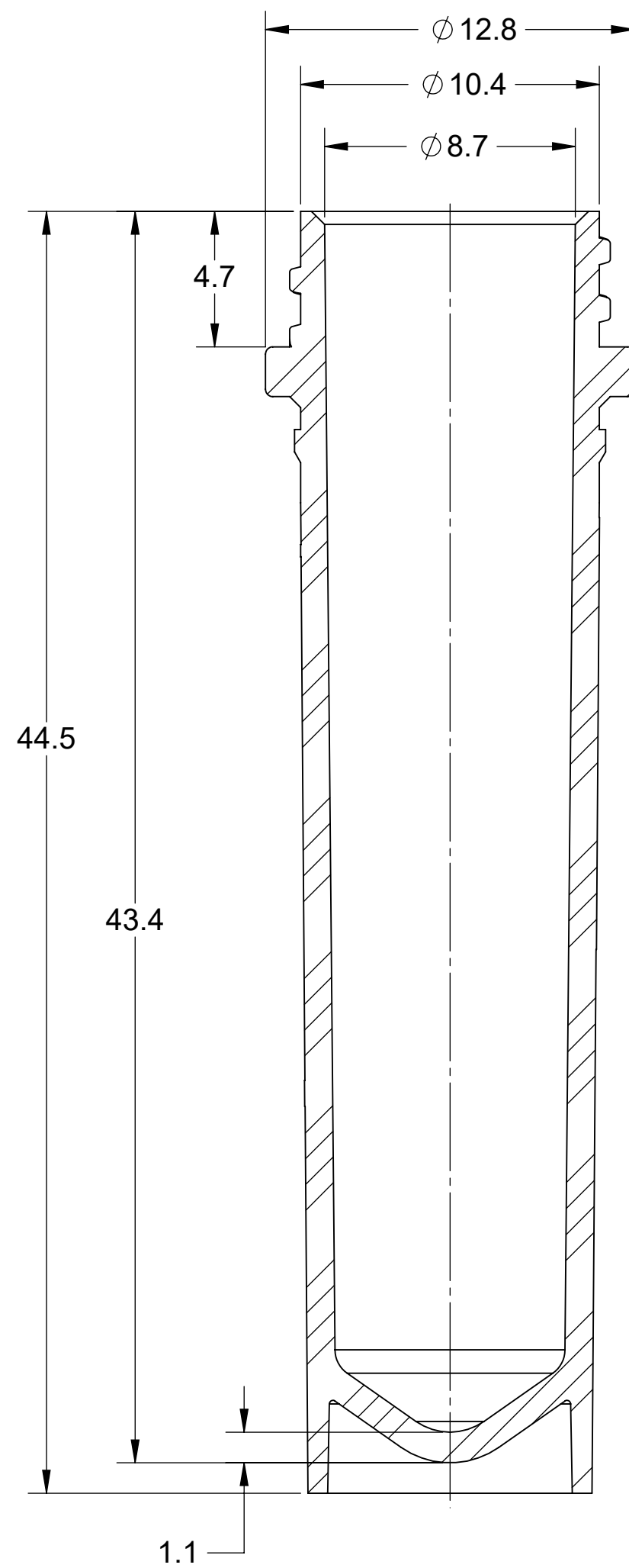
SECTION A-A
