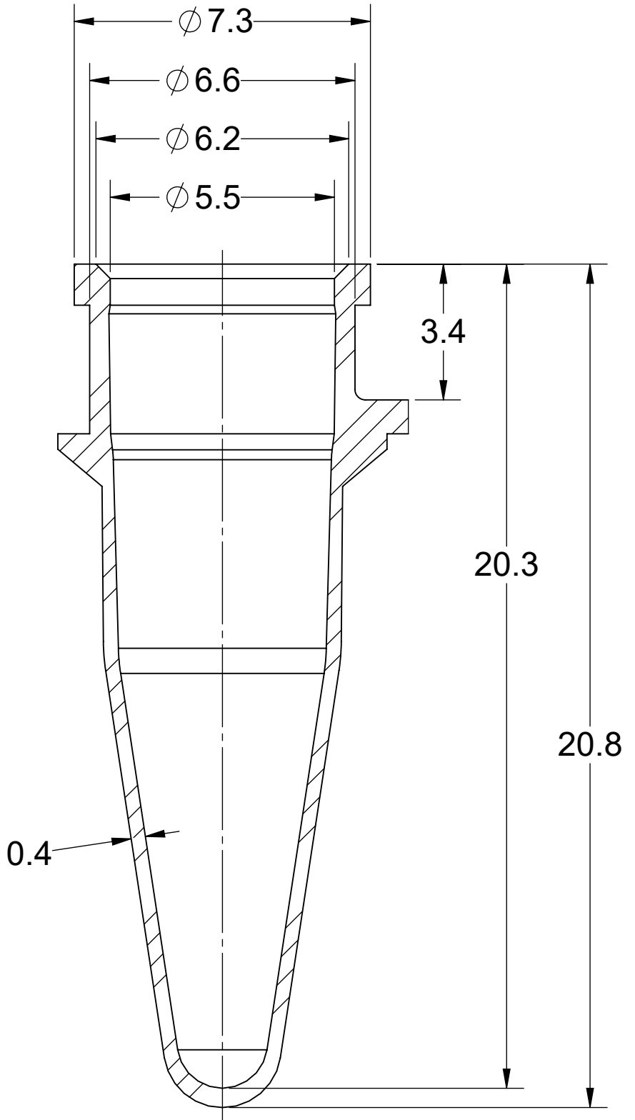
DETAIL B SCALE: 7.5 : 1 TYP
