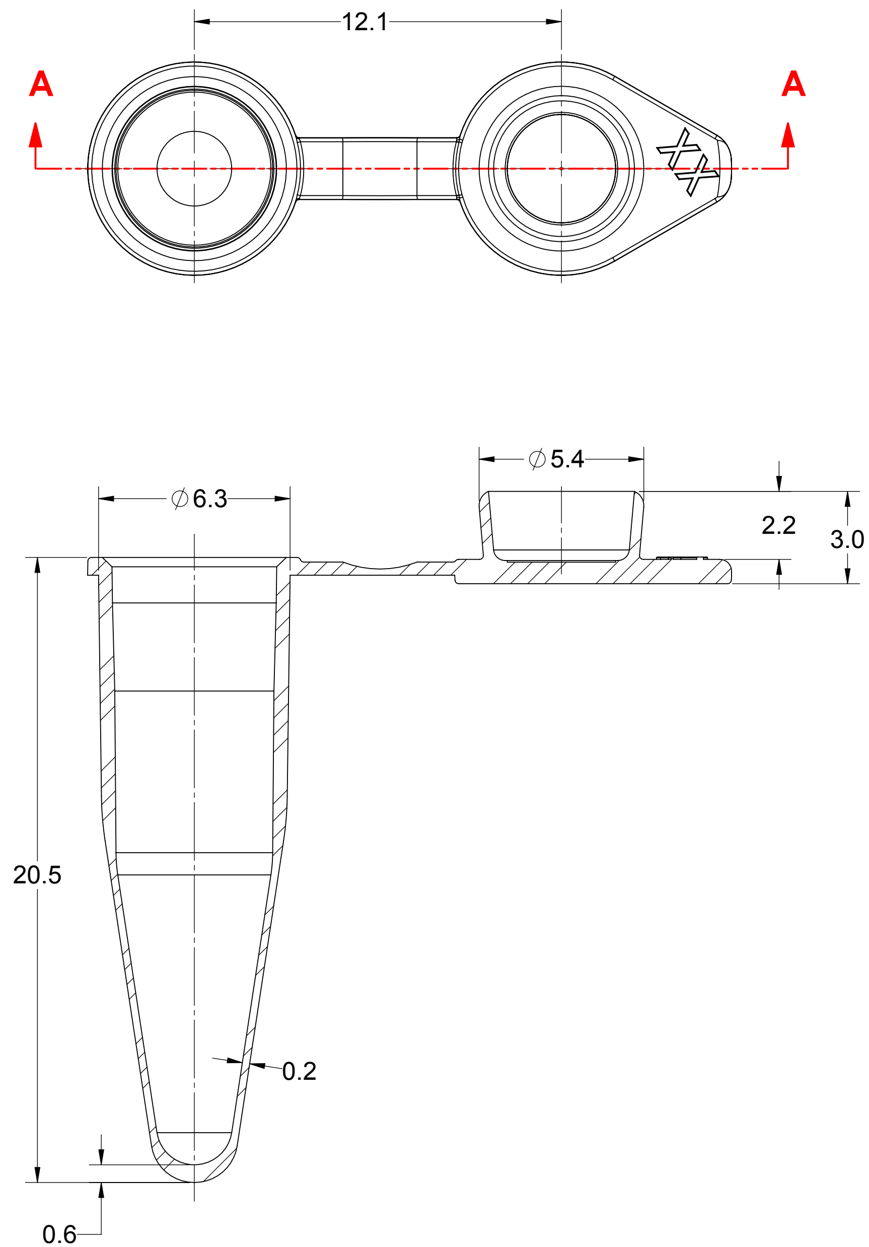
SECTION A-A
