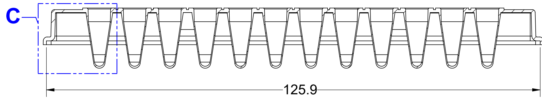
SECTION A-A
