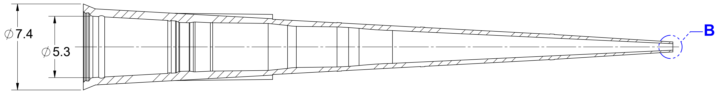
SECTION A-A
