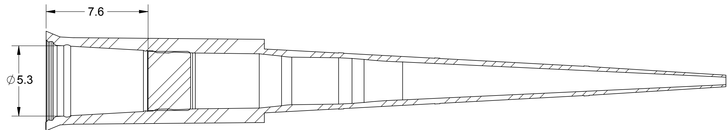
SECTION A-A
