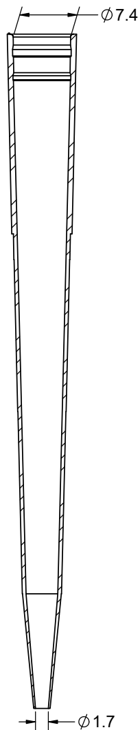
SECTION A-A
