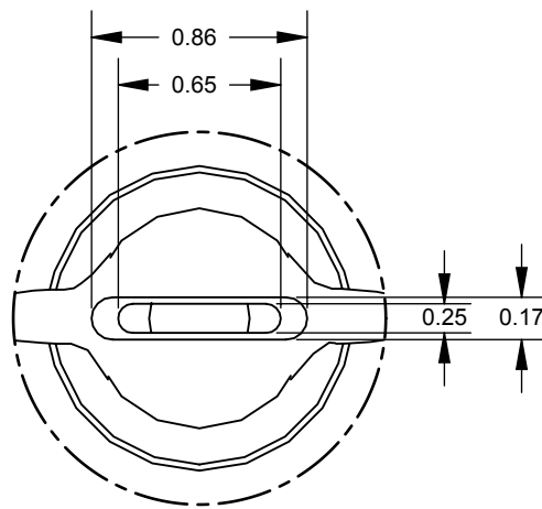
DETAIL B SCALE: 30 : 1
