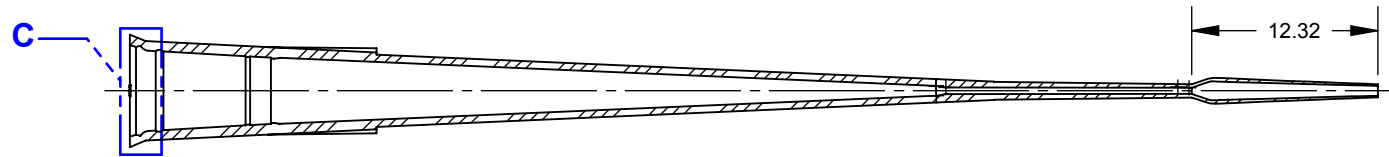
SECTION A-A SCALE: 2 : 1
