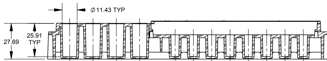
SECTION A-A SCALE: 0.6 : 1
