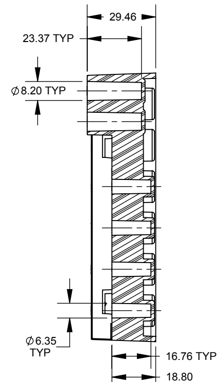
SECTION B-B SCALE: 0.6 : 1
