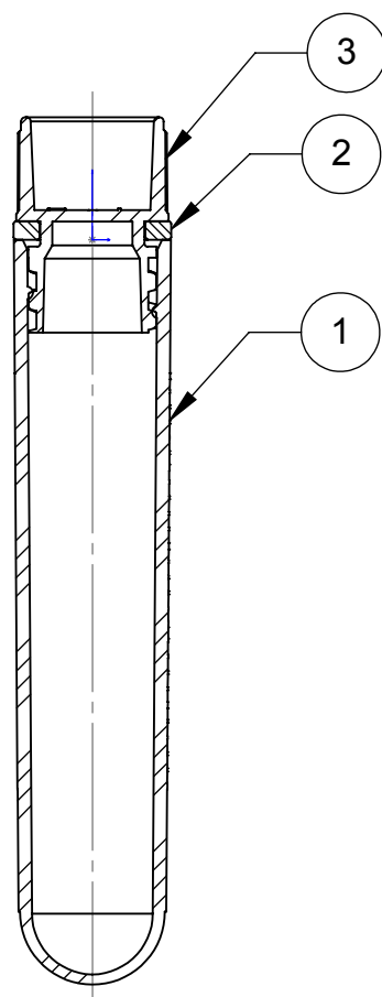
SECTION A-A
