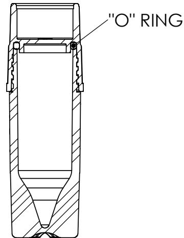
SECTION A-A SCALE 3 : 1
