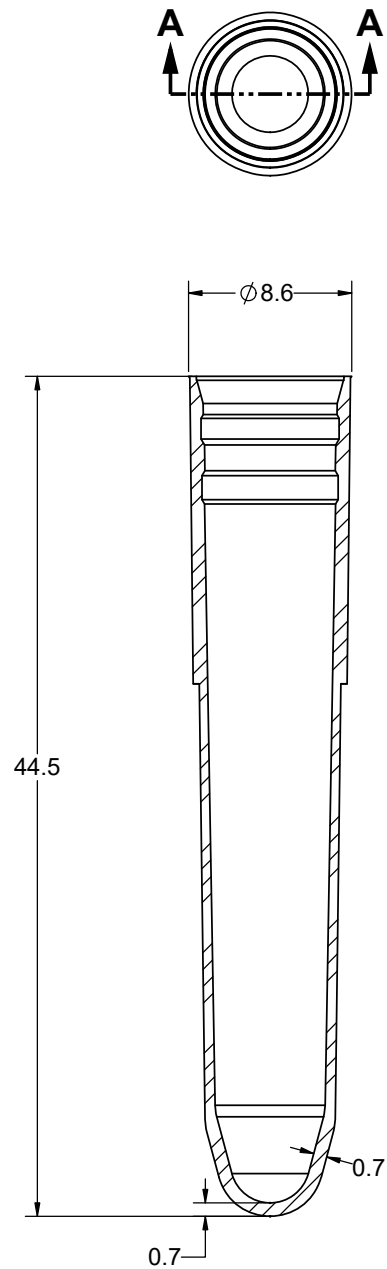
SECTION A-A
