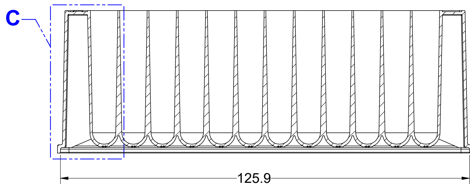
SECTION A-A
