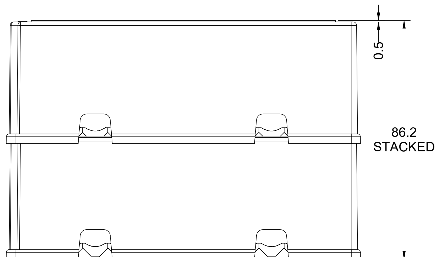
SECTION A-A
